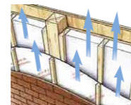
9 家を100年持たせる通気工法
